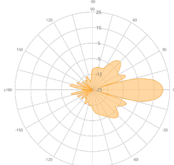
N5-X20 (20 dBi)
