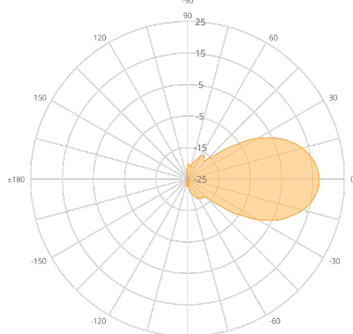
N5-X16 (16 dBi)
